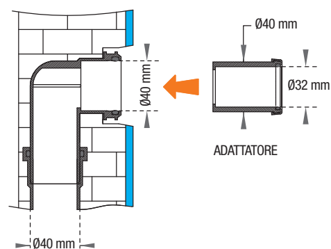
TUBO SENZA IL TAPPO A PERDERE, PRONTO PER RICEVERE IL SIFONE
