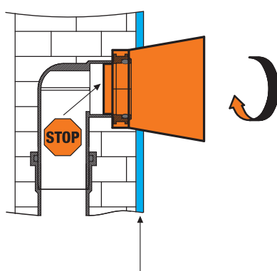
MURO INTONACATO/PIASTRELLATO CON TUBO ANCORA TAPPATO
